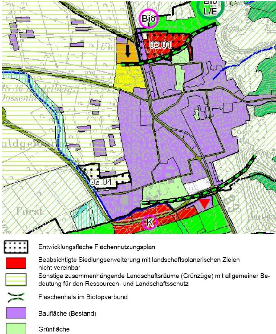
Abbildung 4: Landschaftsplanerischer Konfliktplan
